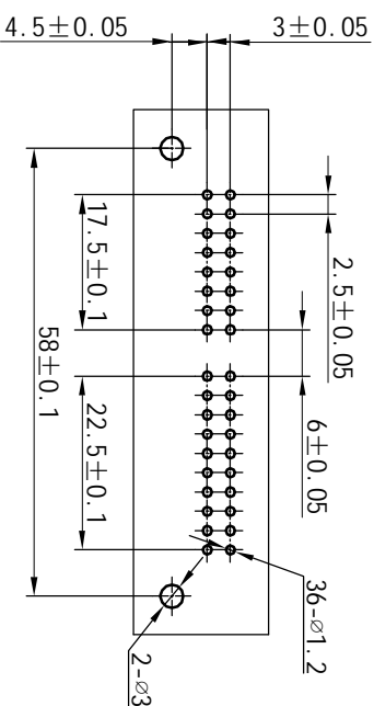
POB板孔位示意图
