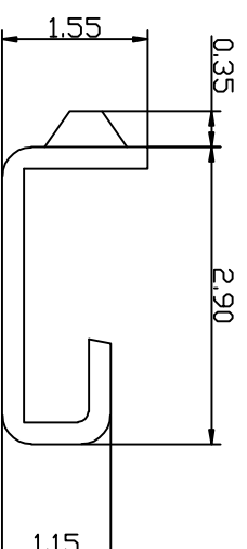
SEC: D-D
