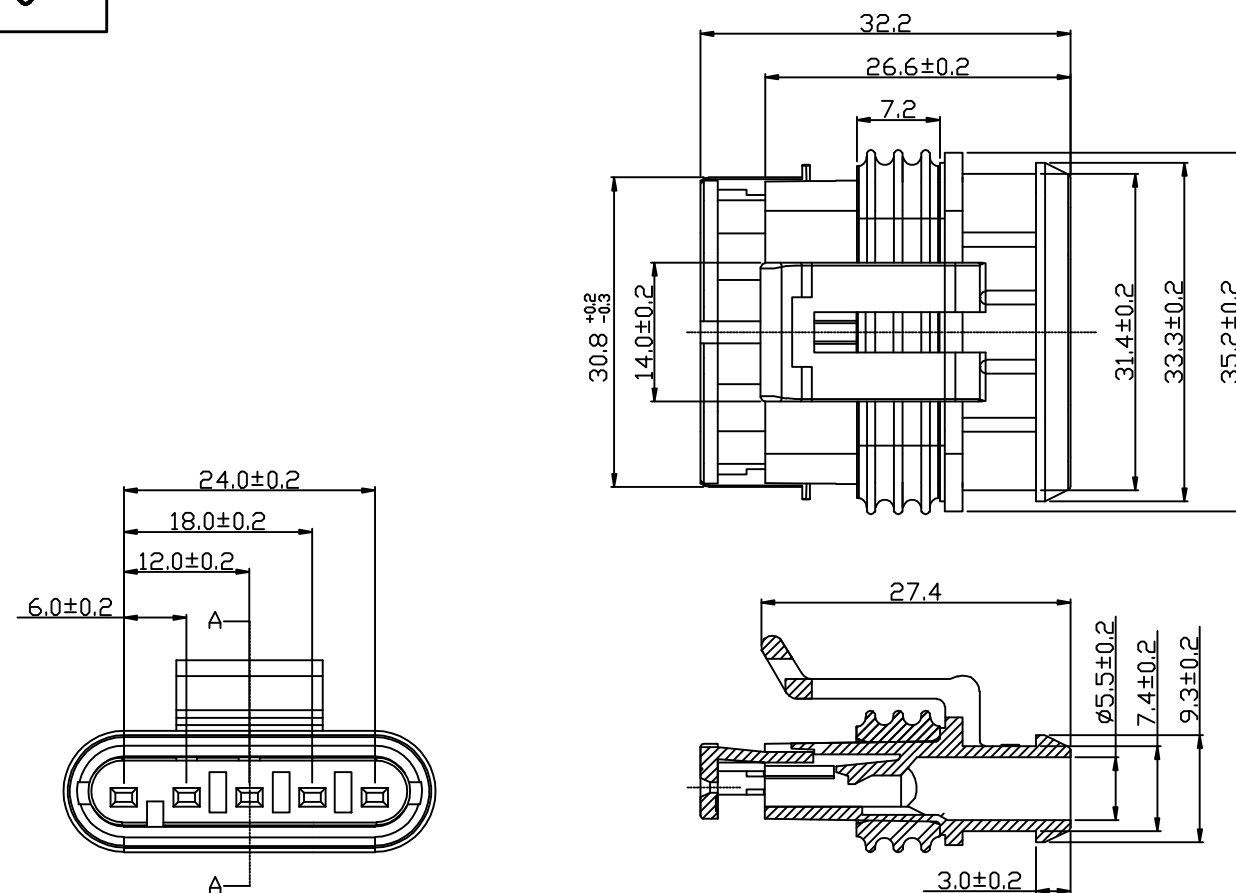
SECTION A-A
