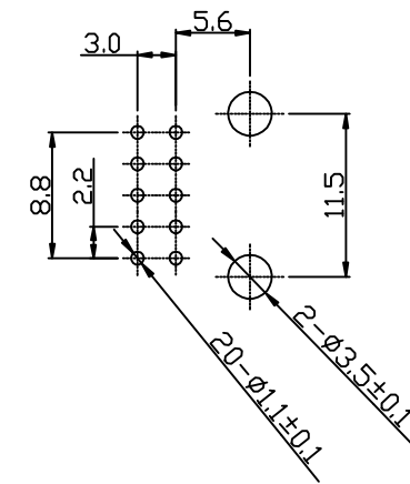
PCB 板孔示意图
