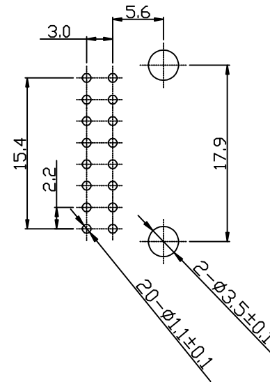
PCB 板孔示意图
