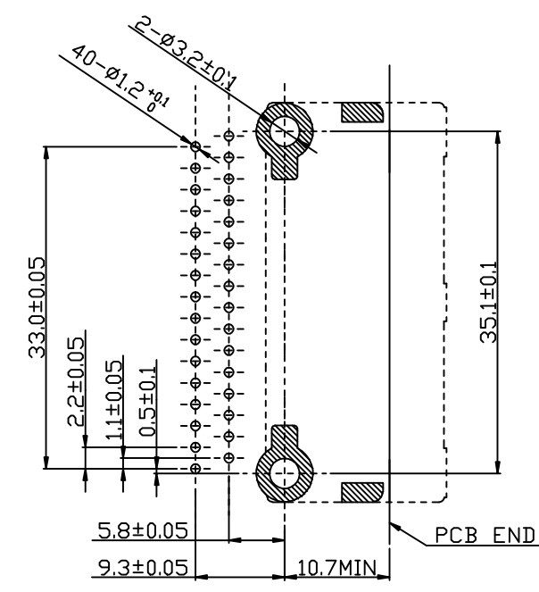
PCB 板孔示意图
