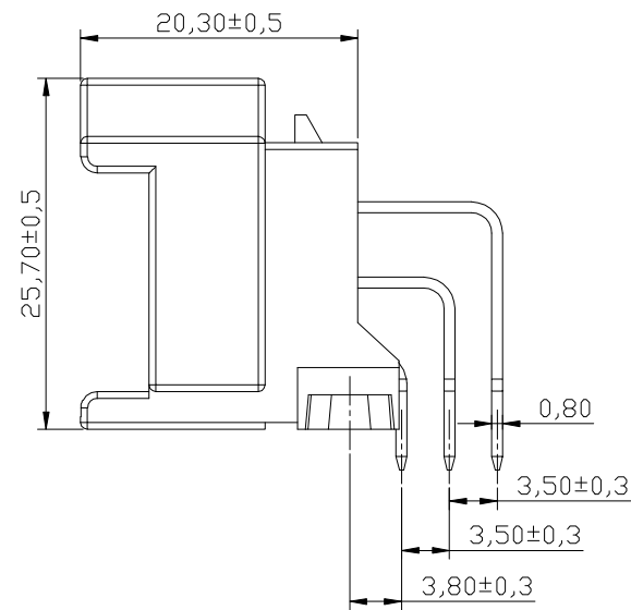
系列尺寸表
